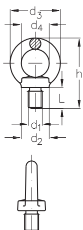
Anneau fileté INOX filetage à droite
