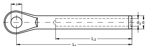
ASS Eye Terminal, Maxi type
